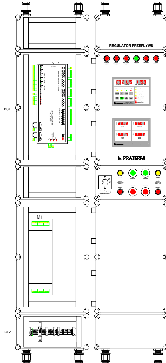
ROZMIESZCZENIE ELEMENTÓW W SZAFIE
